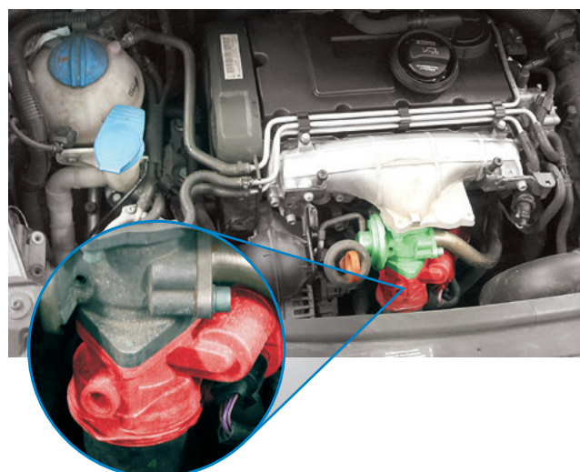
Vue du compartiment moteur du Touran signalé en vert : soupape d'AGR; signalé en rouge : papillon des gaz
